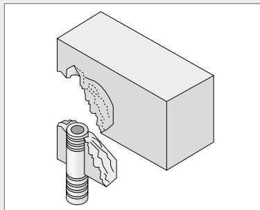
Bruch des Ankergrundes
