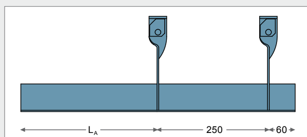
ELMCO–EW, Auskrägung links, ( L_A = Auskrägungslänge)
