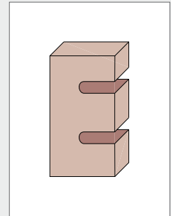
Um den letzten Grenadier im Sturz zu setzen, wird der Stein wie abgebildet eingeschlitz.
