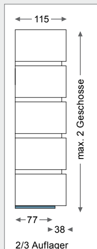
Konsolaufleger und Aufmauerungshöhen für unterschiedliche Ausführungen
