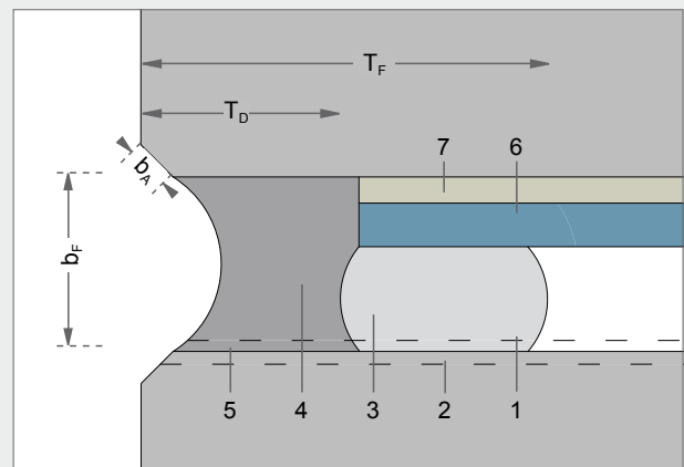
Horizontale Fugenausbildung
