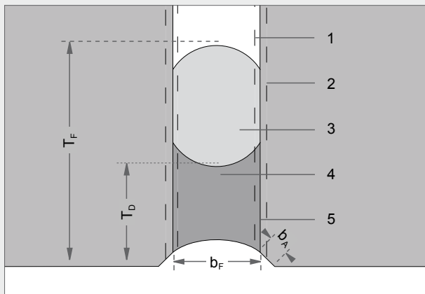
Vertikale Fugenausbildung
